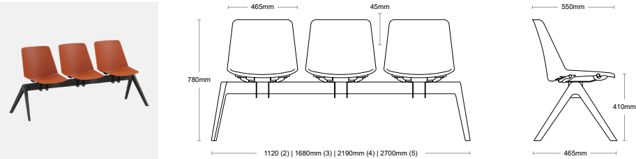
1 Opções de Casco - Shell Options Opciones de casco - Options de coque
