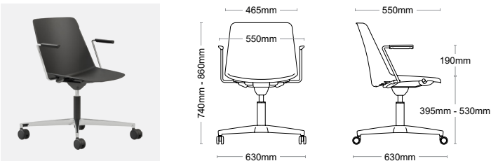
O 4 Hastes rodada - 4 Star base with casters 4 Varillas con ruedas - 4 Tiges avec roulettes
