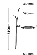
F Piramidal c/ Apoio de Braço - Pyramidal with Armrest Piramidal con reposabrazos - Pyramidal avec accoudoir
