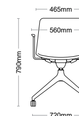
H Piramidal Rodada c/ Apoio de Braço - Pyramidal with casters and armrest Piramidal con ruedas y reposabrazos - Pyramidal avec roulettes et accoudoir
