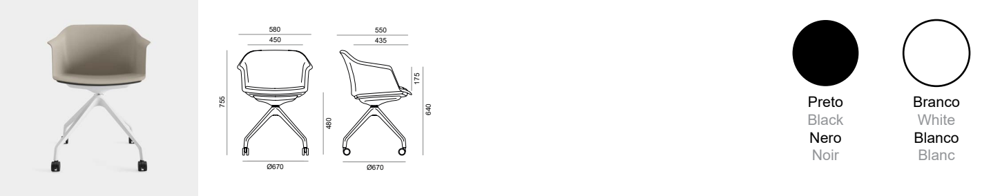
H 4 Hastes rodada - 4 Star base w/ casters - 4 Varillas con ruedas - 4 Tiges avec roulettes
