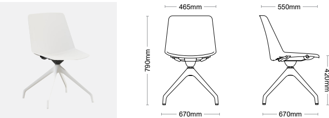
M Piramidal (polipropileno) - Pyramidal (polypropylene) Piramidal (polipropileno) - Pyramidal (polypropylène)
