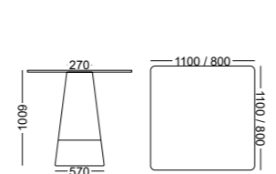
C Mesa alta c/ tampo quadrado em aglomerado (melamina), base estodada. High table w/ square top in chipboard (melamine coated), upholstered base. Mesa alta c/ tapa cuadrada en aglomerado (melamina), base tapizada. Table haute a/ plateau carré en aggloméré (mélaminé), piétement rembourré.
