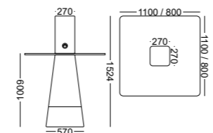
D 2 Com 4 Tomada e 4 USB nas quatro faces do módulo central. With 4 Socket and 4 USB in the four sides of the centre module. Con 4 Enchufe y 4 USB en los cuatro lados del módulo central. Avec 4 Prise et 4 USB sur les quatre côtés du module central.
