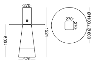
B 1 Com 2 Tomada e 2 USB em duas faces opostas do módulo central. With 2 Socket and 2 USB on two opposite sides of the central module. Con 2 Enchufe y 2 USB en dos lados opuestos del módulo central. Avec 2 Prise et 2 USB sur deux côtés opposés du module central.
