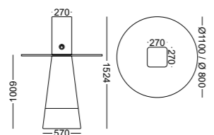
B 2 Com 4 Tomada e 4 USB nas quatro faces do módulo central. With 4 Socket and 4 USB in the four sides of the centre module. Con 4 Enchufe y 4 USB en los cuatro lados del módulo central. Avec 4 Prise et 4 USB sur les quatre côtés du module central.
