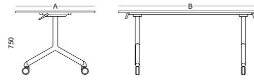
Mesa rebatível com sistema hidráulico - Folding table with hydraulic system - Mesa plegable con sistema hidráulico - Table pliante avec système hydraulique Patilha de ajuste - Adjustment tab - Pestaña de ajuste - Onglet de réglage
