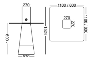
D 1 Com 2 Tomada e 2 USB em duas faces opostas do módulo central. With 2 Socket and 2 USB on two opposite sides of the central module. Con 2 Enchufe y 2 USB en dos lados opuestos del módulo central. Avec 2 Prise et 2 USB sur deux côtés opposés du module central.
