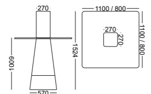
D Mesa alta c/ módulo central, tampo quadrado em aglomerado (melamina), base estodada. High table w/ central module, square top in chipboard (melamine coated), upholstered base. Mesa alta c/ módulo central, tapa cuadrada en aglomerado (melamina), base tapizada. Table haute a/ plateau carré aggloméré (mélaminé), piétement rembourré.
