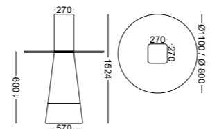
B Mesa alta c/ módulo central, tampo redondo em aglomerado (melamina), base estodada. High table w/ central module, round top in chipboard (melamine coated), upholstered base. Mesa alta c/ módulo central, tapa redonda en aglomerado (melamina), base tapizada. Table haute a/ plateau rond aggloméré (mélaminé), piétement rembourré.
